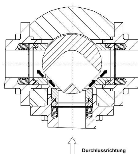
Bild 16 „Mit Überschneidung“
