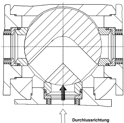
Bild 15 „Überschneidungsfrei“
