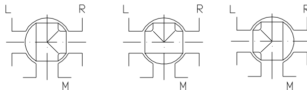
Bild 12 T-Bohrung
